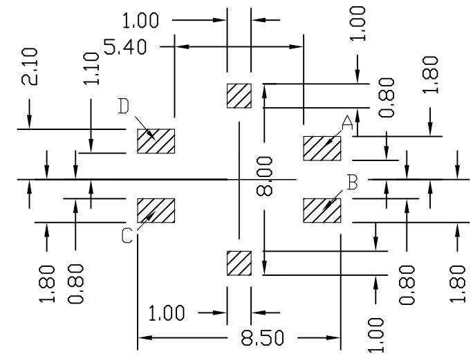
P.C.B. LAYOUT
