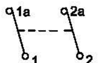
CIRCUIT DPST
