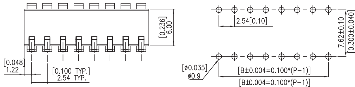
P.C.B. LAYOUT
