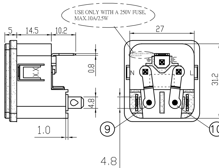
剖面圖 A-A
