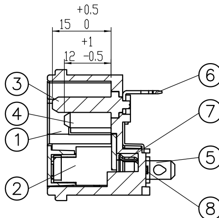
剖面圖 A-A
